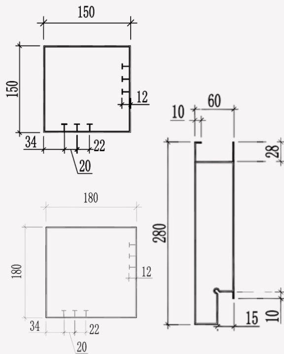
COLONNE COLUMN
